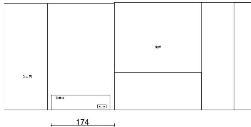
A-4 進門玄關櫃
