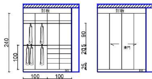
D-2 次臥2 衣櫃
