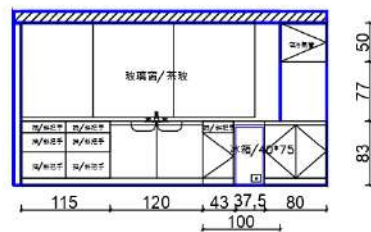
B-1 流理台立面
