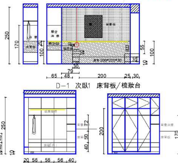
D-2 次臥1 衣櫃
