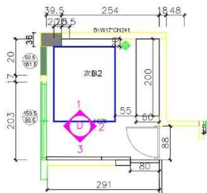
D-1 次臥2 床頭
